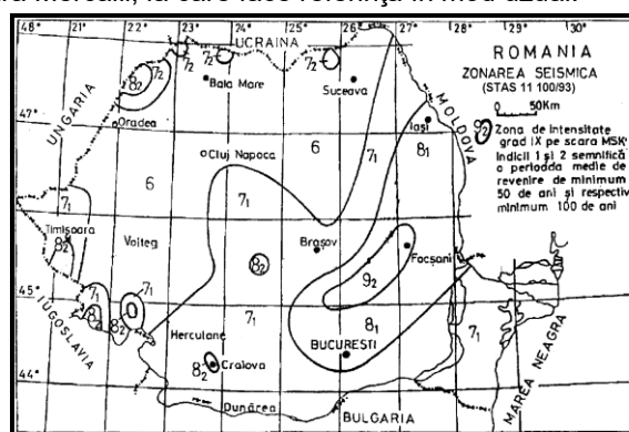
Fig. 2. a. Zonarea seismică a teritoriului României – intensități pe scara MSK , conf. SR 11100 – 1: 93 Zonarea seismică. Macrozonarea teritoriului României (indicele 1 indică o perioadă medie de revenire de minimum 50 de ani iar indicele 2 indică o perioadă medie de revenire de minimum 100 de ani a intensităților respective)
